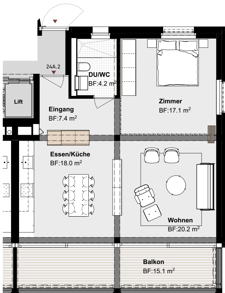
24A.2 2.5 ZIMMER-WOHNUNG HNF= 67.1 m 2
