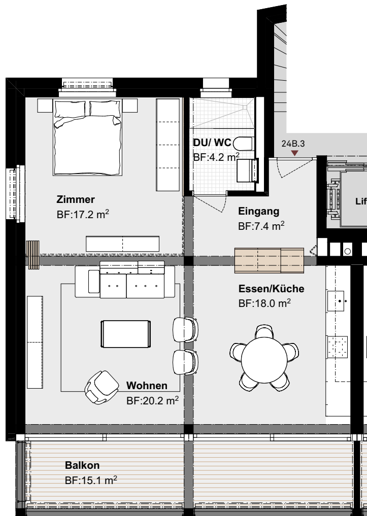
24B.3 2.5 ZIMMER-WOHNUNG HNF= 67.1 m 2
